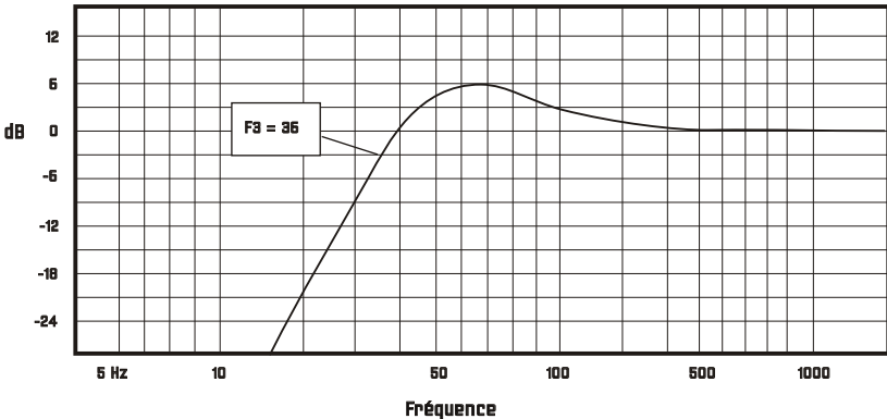
Réponse en amplitude ELW1514P (dB/Hz)
