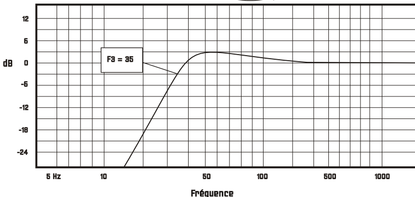
Réponse en amplitude ELW1214P (dB/Hz)
