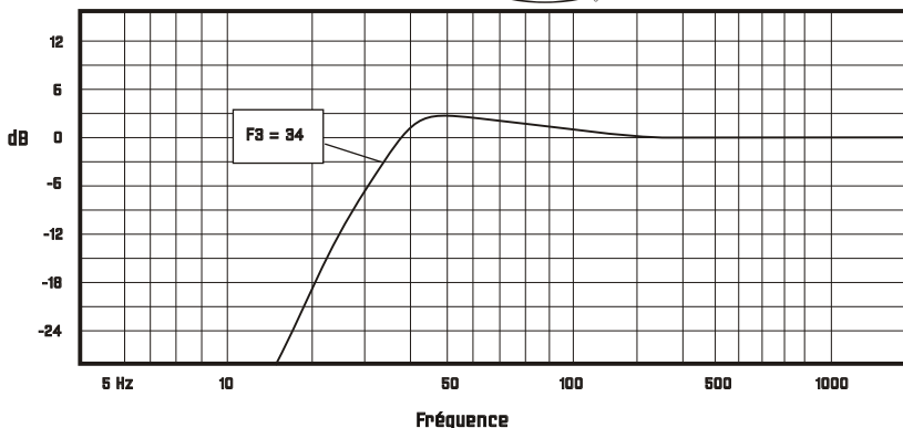
Réponse en amplitude ELW1014P (dB/Hz)
